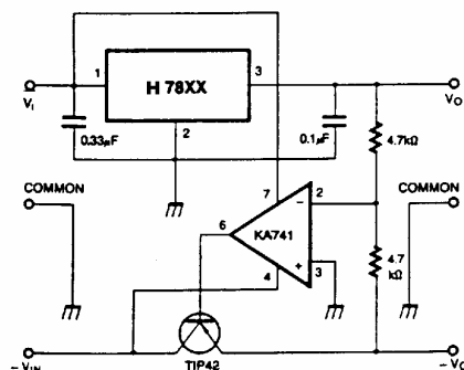
图 10、跟踪稳压器
