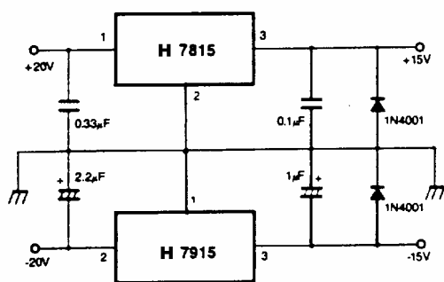
图 11、分离电源( \pm 15V-1A )
